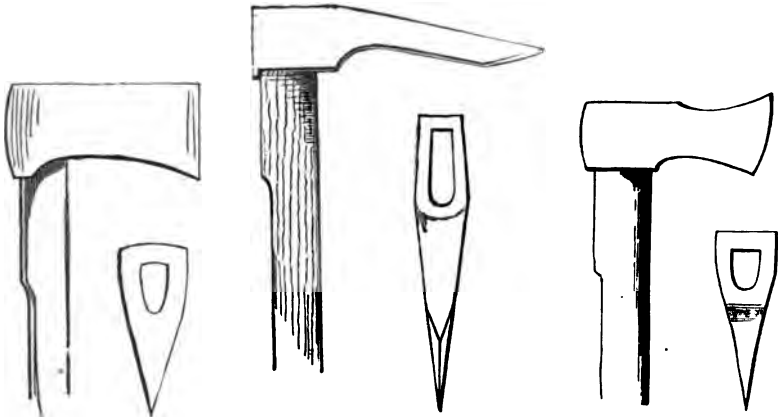
Fig. 127. The Prague cleaving-axe.
